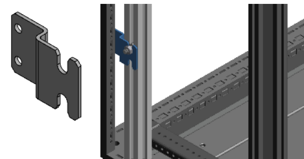
MBS.070 Adaptionswinkel TS8
