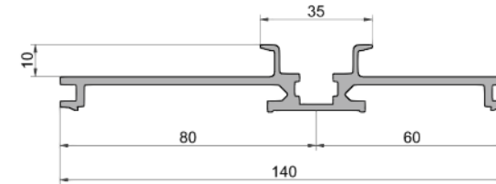
Gleitmuttern
