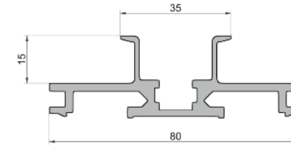
Gleituttern
